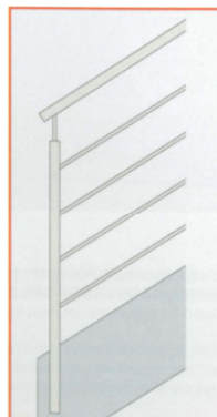
ROMA „Q“ Mit quadratischen Pfosten und 4 parallelen Gurten in Edelstahl und Holz-Handlauf
