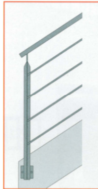
Modell GSP-S Mit T-Profil-Pfosten aus Stahl, 4 parallelen Edelstahlseilen und Holz-Handlauf
